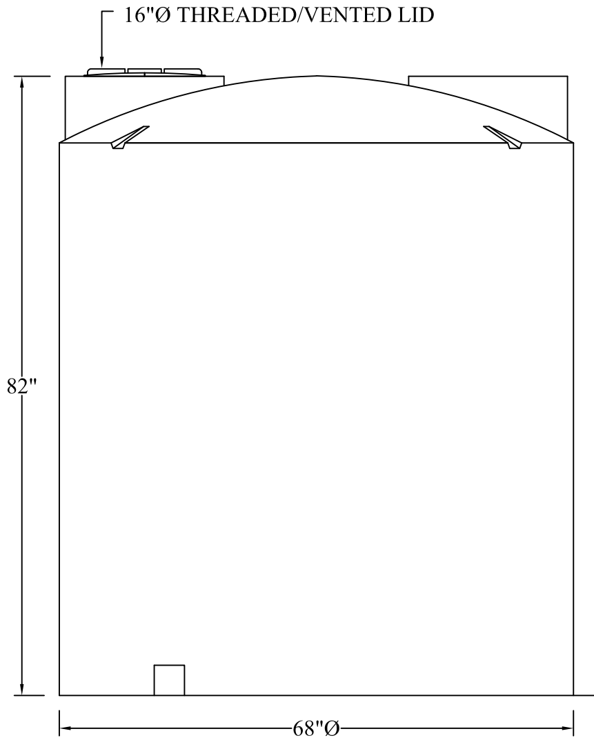
ELEVATION
