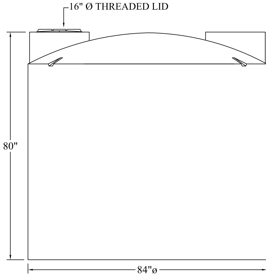
ELEVATION
